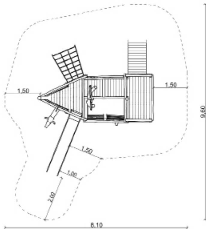
Draufsicht mit Mindestraum
