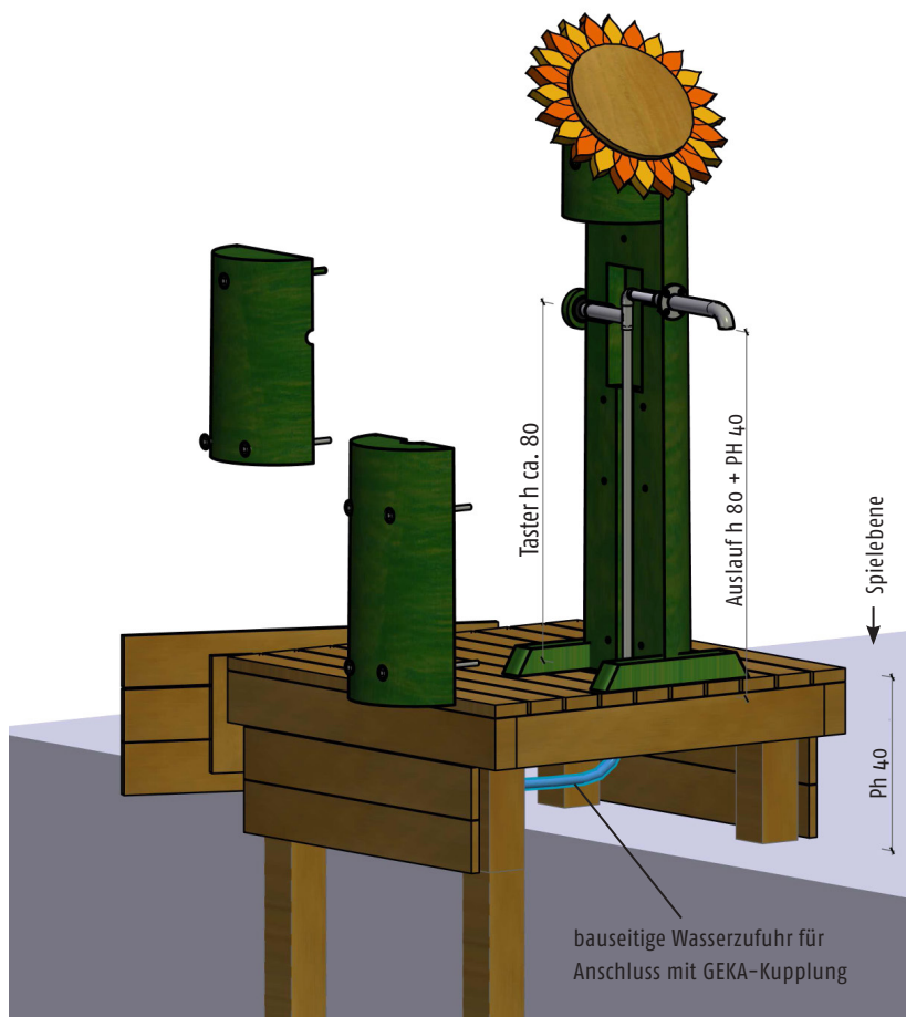
8.30.5.3.3 Wasserstelle »Blume« Anschluss unter Podestfläche
