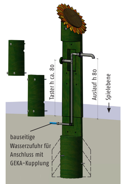
8.30.5.3.1 Wasserstelle »Blume« Anschluss unter OK Spielebene
