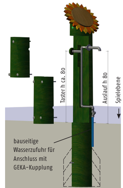
8.30.5.3.2 Wasserstelle »Blume« Anschluss über OK Spielebene (nur für nichtöffentliche Bereiche)
